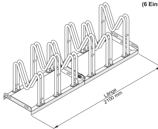
Modell Harlekin 6 (6 Einstellplätze)
