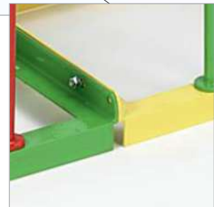
Grundrahmen aus Winkelstahl (35x35 mm) mit abgerundeten Ecken - keine Verletzungsgefahr. Bodenbefestigung und Reihen- verbindung möglich.
