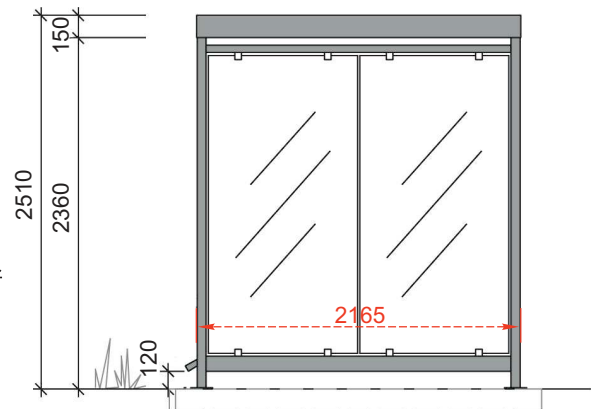
Seitenansicht
