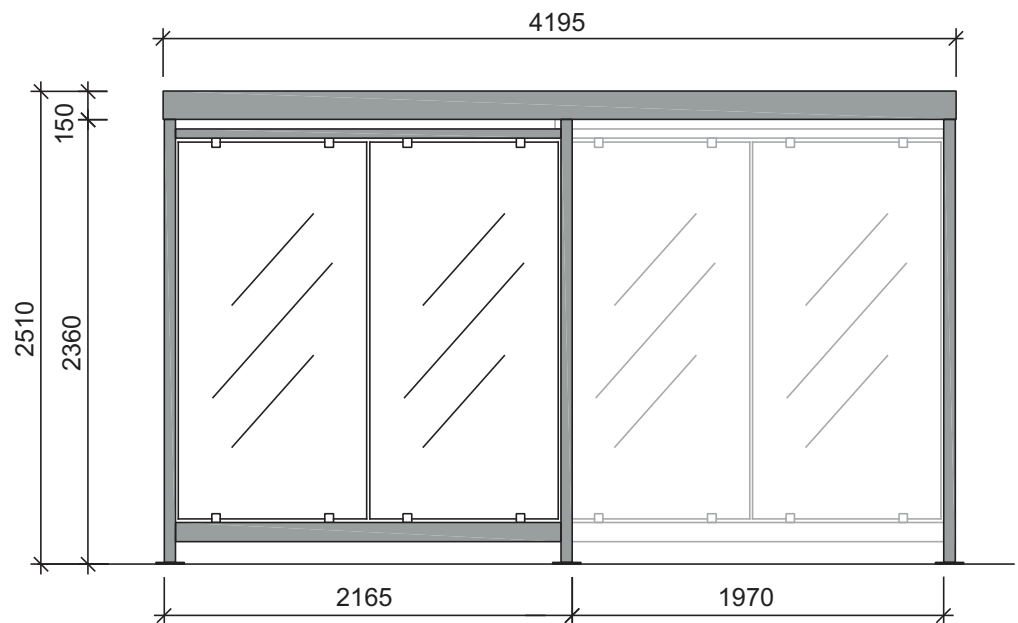
Vorderansicht
